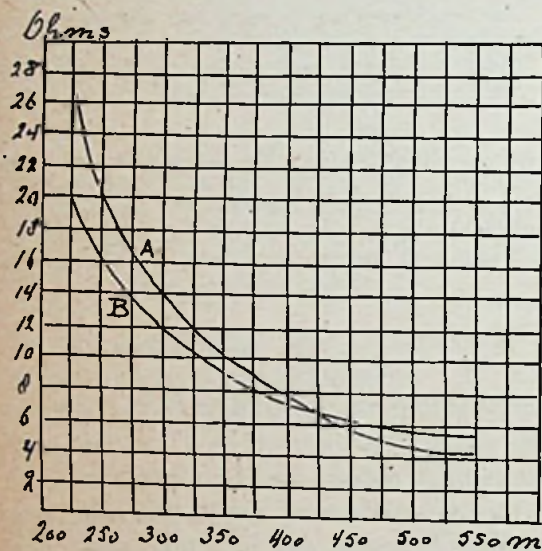
Fig. 6. De hoogfrequentie weerstand van twee verschillende spoelen voor de korte omroepgolven. De weerstanden zijn gemeten met inbegrip der normale diëlectrische verliezen. A. Spoel met diameter 75 mm, 72 windingen litzedraad 27/47. Zelfinductie 260 \mu H. B. Spoel met diameter 50 mm, 80 naast elkaar gelegde windingen van draad no. 26 SWG met dubbel katoen Zelfinductie 200 \mu H.
