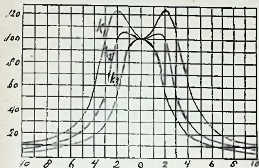
Fig. 2. Dubbele pieken ontstaan bij enigszins sterke koppeling tusschen twee gelijk afgestemde kringen. De horizontale verdeling geeft het aantal kilo Hertz buiten afstemming. Verticaal een willekeurige sterkte schaal; k_1 sterke koppeling, k_2 middelmatige en k_3 zwakke koppeling.
