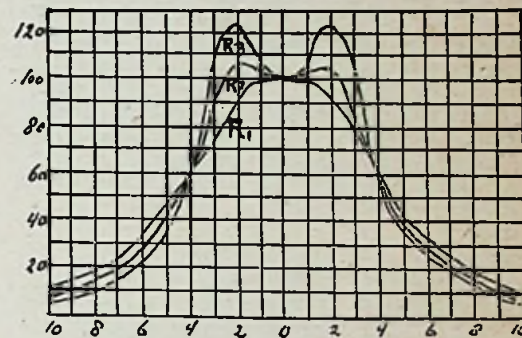
Fig. 5. Invloed van den kringweerstand op den vorm der afstemkromme van 2 kringen met gelijkblijvende koppeling. De horizontale verdeling geeft het aantal kHz buiten afstemming. R_1 groote weerstand, R_2 kleinere en R_3 kleinste weerstand.
